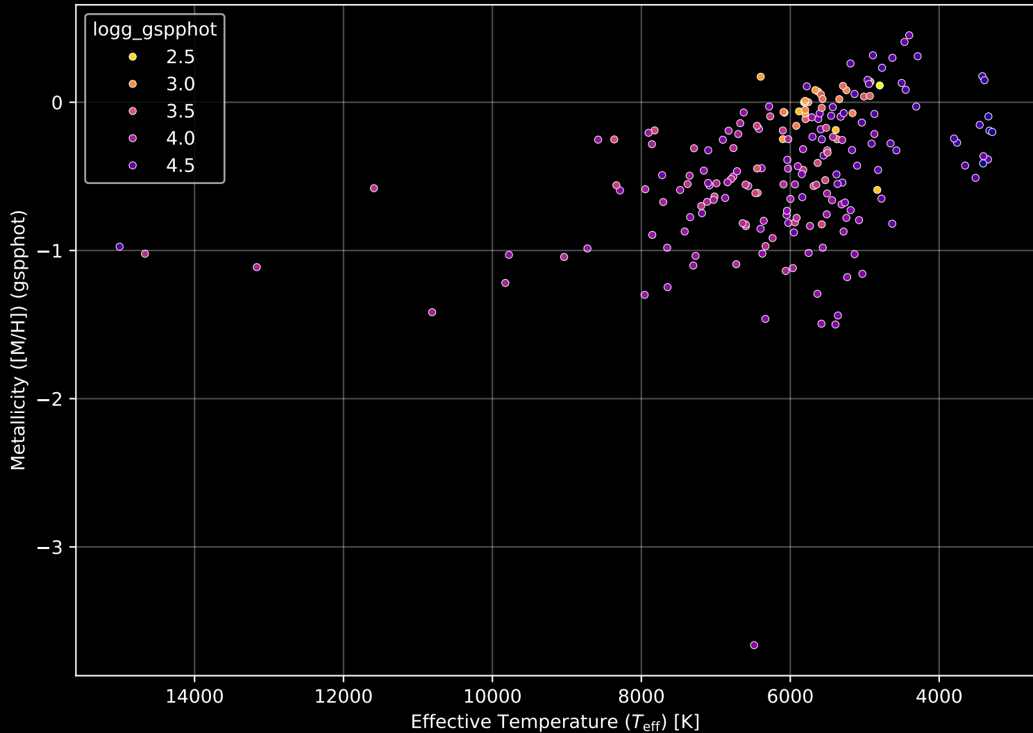
APOGEE DR17 Field: [K2_C13_175-10_btx] Stellar Population Parameters (n= 204)
